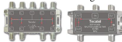
fig. 4: repartidores varias salidas
